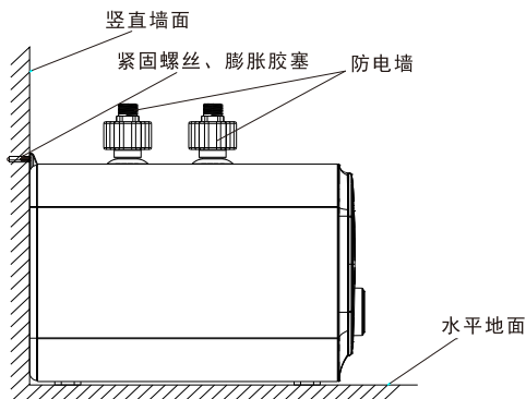
安装示意图
